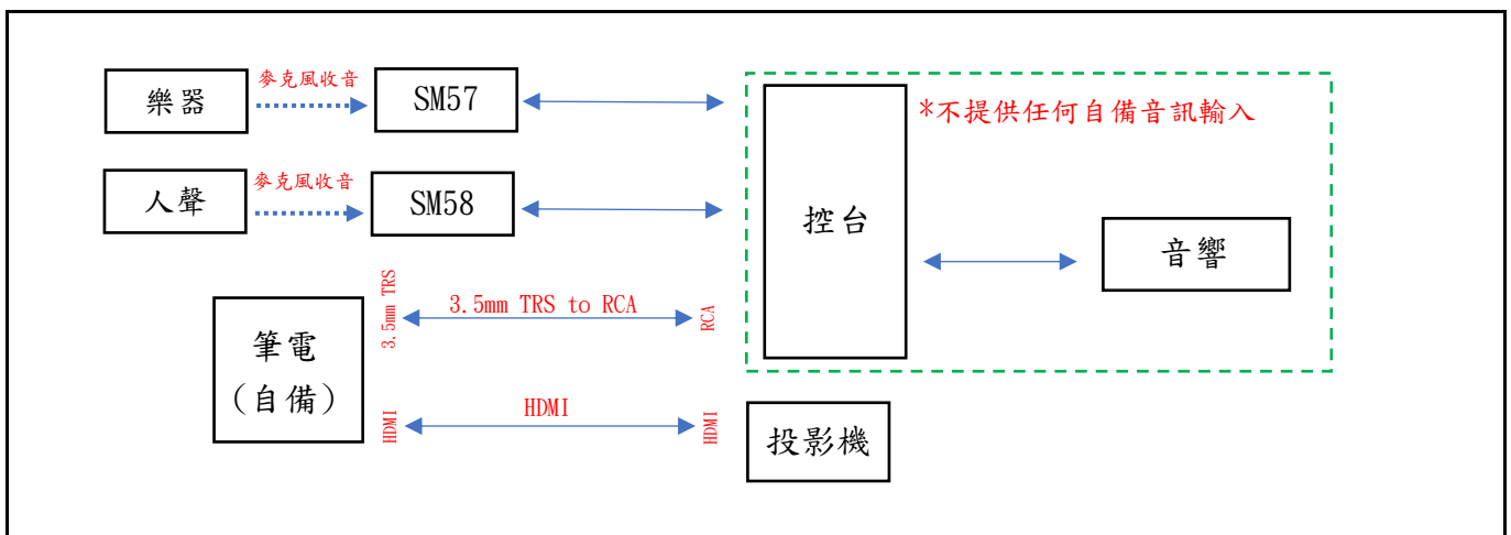
↑考場內設備線路示意圖，供參閱↑
